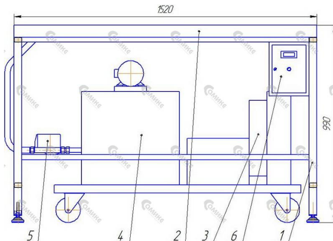
Рис. 1 Стол охлаждающий кондитерских масс СОКМ-30
